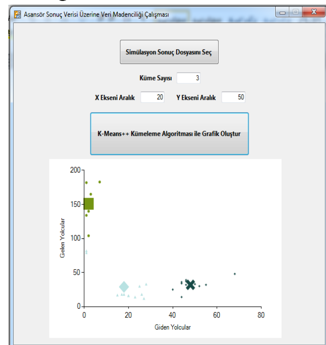
Şekil 4: Ek program görüntüsü.
