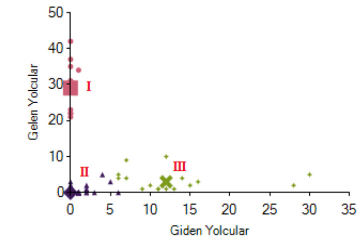
Şekil 6: Okulun asansör trafiği için kümeleme sonucu
