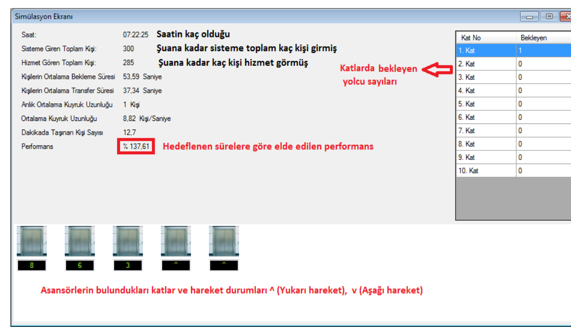
Şekil 2: Simülasyon ekranı.
